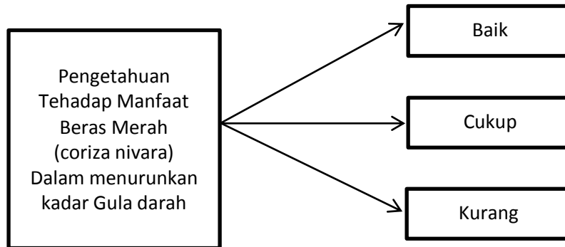
Gambar 2.1 Kerangka Konsep
